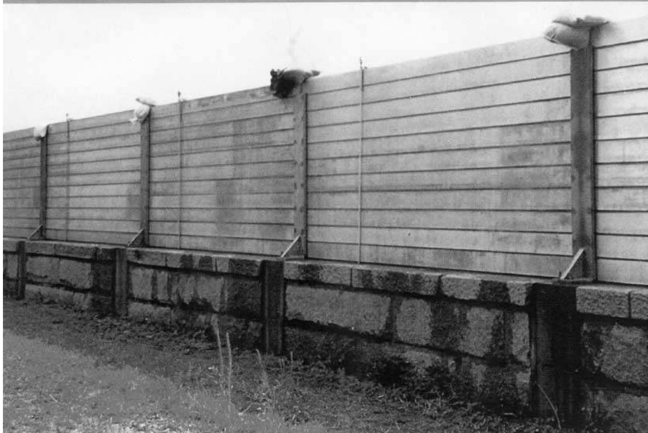
Für den Ortsteil von Marbach sind mobile Hochwasserschutzwände, wie sie schon 2002 in Krems zum Einsatz kamen, geplant.
